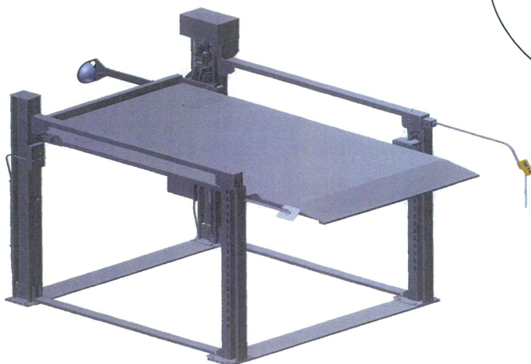
類型 2 : ピット二段(三段)昇降式
